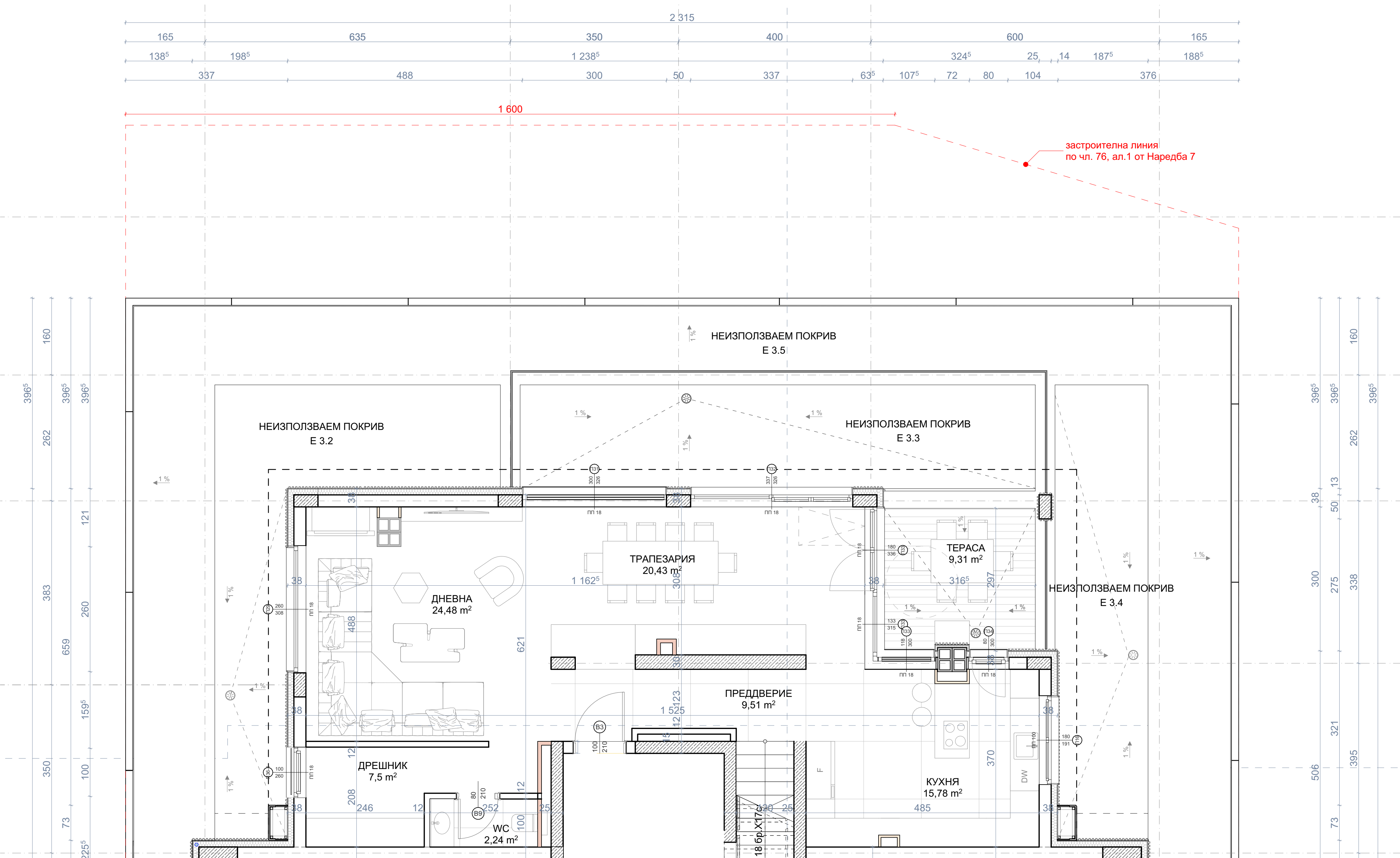
АПАРТАМЕНТ 11 - ПЪРВО НИВО
